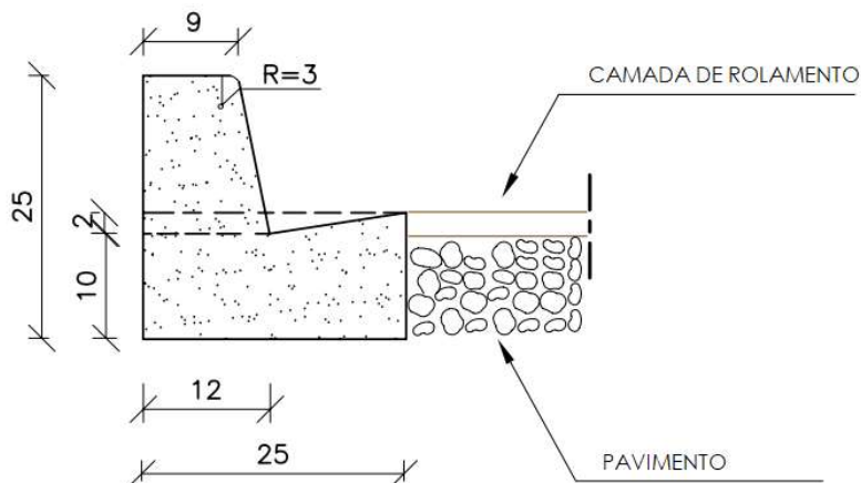
Figura 03 – Meio-fio e sarjeta do Tipo 2 do Álbum de Projetos-Tipo do DER/PR.
