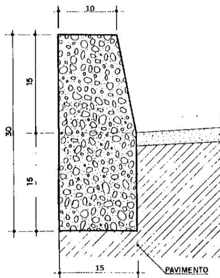
Figura 01 – Meio-fio para canteiros centrais conforme projeto.
