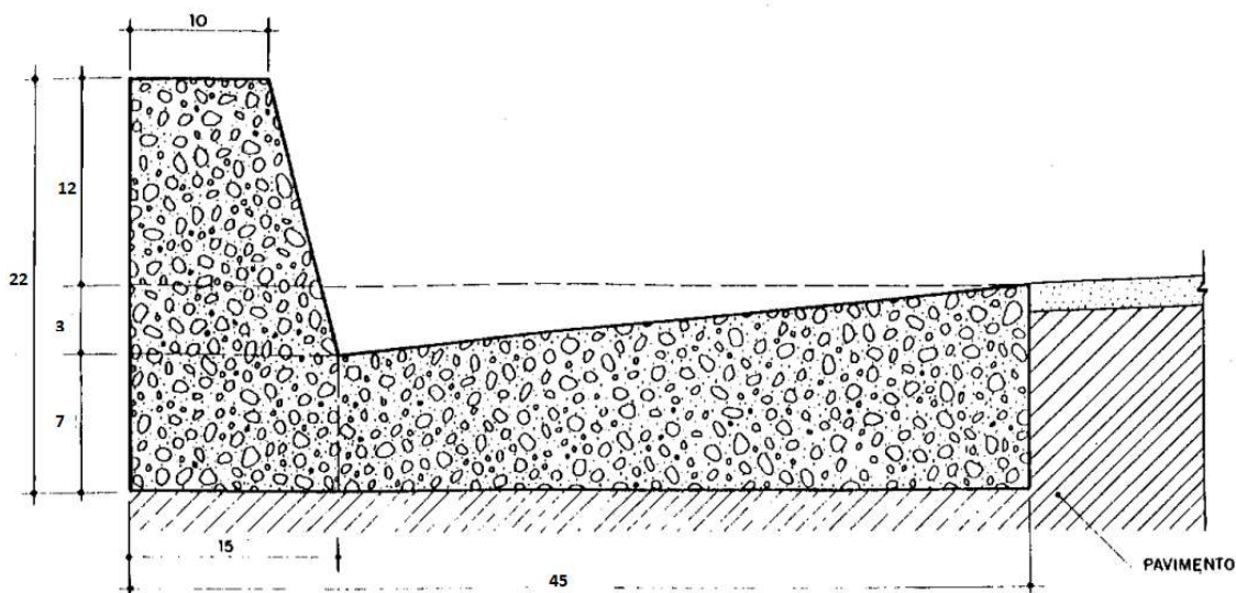
Figura 02 – Meio-fio e sarjeta para calçadas laterais conforme projeto.
